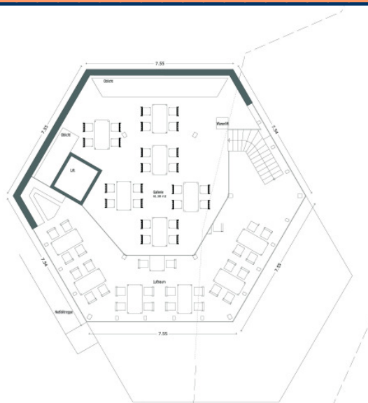
Grundriss Dachgeschoss / Galerie
