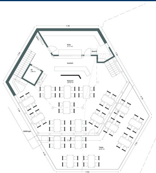
Grundriss 2 Obergeschoss
